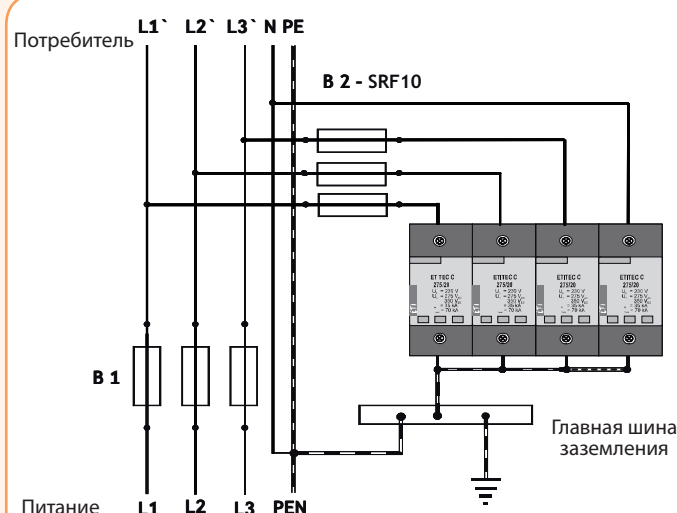
Пример монтажа ограничителей перенапряжения, защищённых предохранителями типа SRF (B2)
